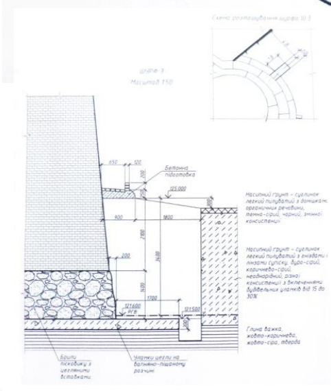
Проект комплексних протизсувних, протиаварійних та реставраційних заходів по підпірній стіні Дебоскета у Києво-Печерській лаврі (частково реалізовано);
