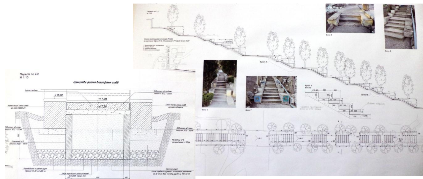
Проект комплексних реставраційних робіт на садибі Жуковського у Кучук-Кої, АР Крим. Сходи Якова (у процесі реалізації);
