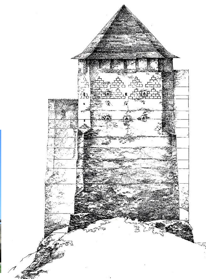
Комплекс реставраційних робіт по фортеці у м. Хотин, Чернівецької обл.. Південна (Візна) та Північна башти (у процесі реалізації);
